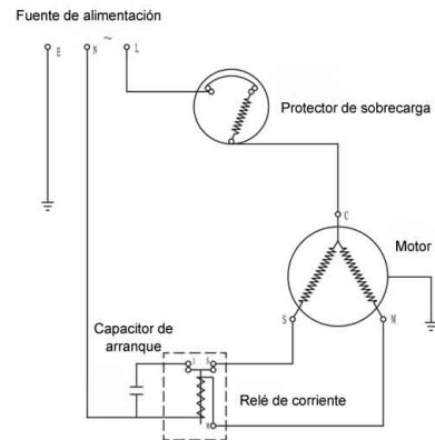
DIAGRAMA ELECTRICO
