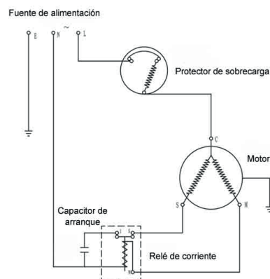
DIAGRAMA ELECTRICO
