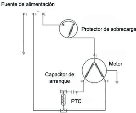
DIAGRAMA ELECTRICO
