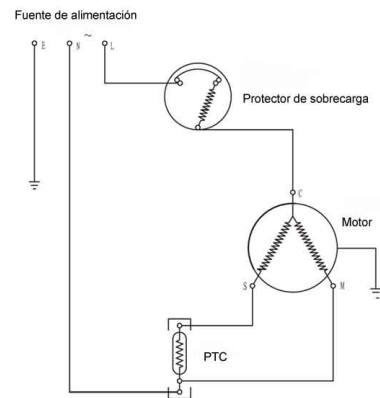
DIAGRAMA ELECTRICO
