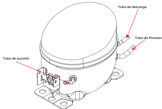
DIAGRAMA DE LINEAS
