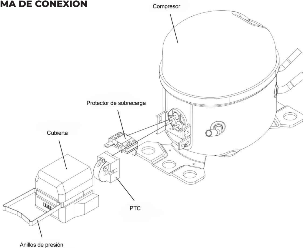
DIAGRAMA DE CONEXIÓN
